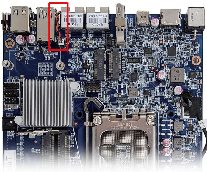
Foto: Position der Knopfzellen-Batterie und des Anschlusses auf dem Mainboard.
