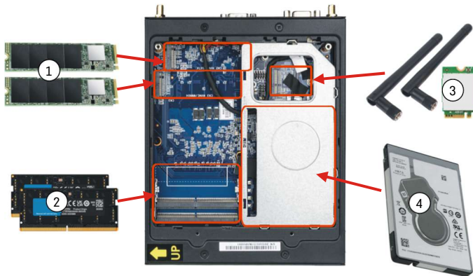
Shuttle XPC slim Barebone DS50U mit geöffnetem Gehäuse
