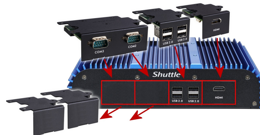
Vue avant (exemple de configuration) Tôles de recouvrement peuvent être remplacés par des ports d'E/S en option
